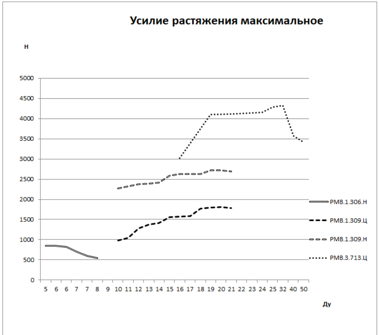
Рис. 4. Сравнительная диаграмма, максимального усилия растяжения.
